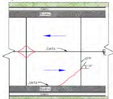
Figura 5. Vista en planta: Grieta de Esquina
