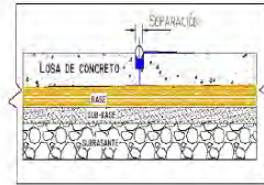
Figura 12. Deterioro del Sello
