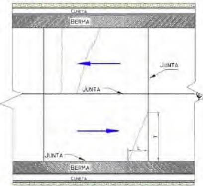
Figura 7. Vista en Planta de las Grietas Transversales.
