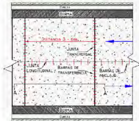
a. Vista en planta
