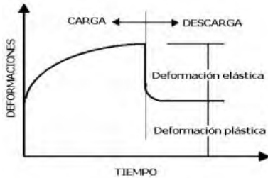
Figura 2. Comportamiento de materiales viscoelásticos.
