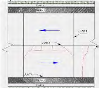
Figura 9. Características de las grietas en bloque
