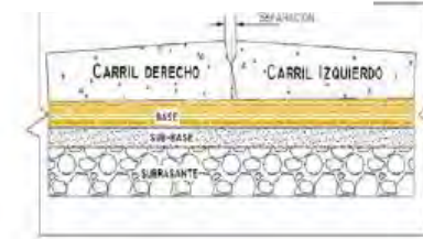
b. Vista en perfil: Detalle Separación de Juntas Longitudinales
