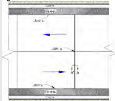
a. Vista en planta. Escalonamiento Junta Transversal.
